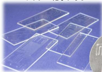
マイクロ化学チップ
